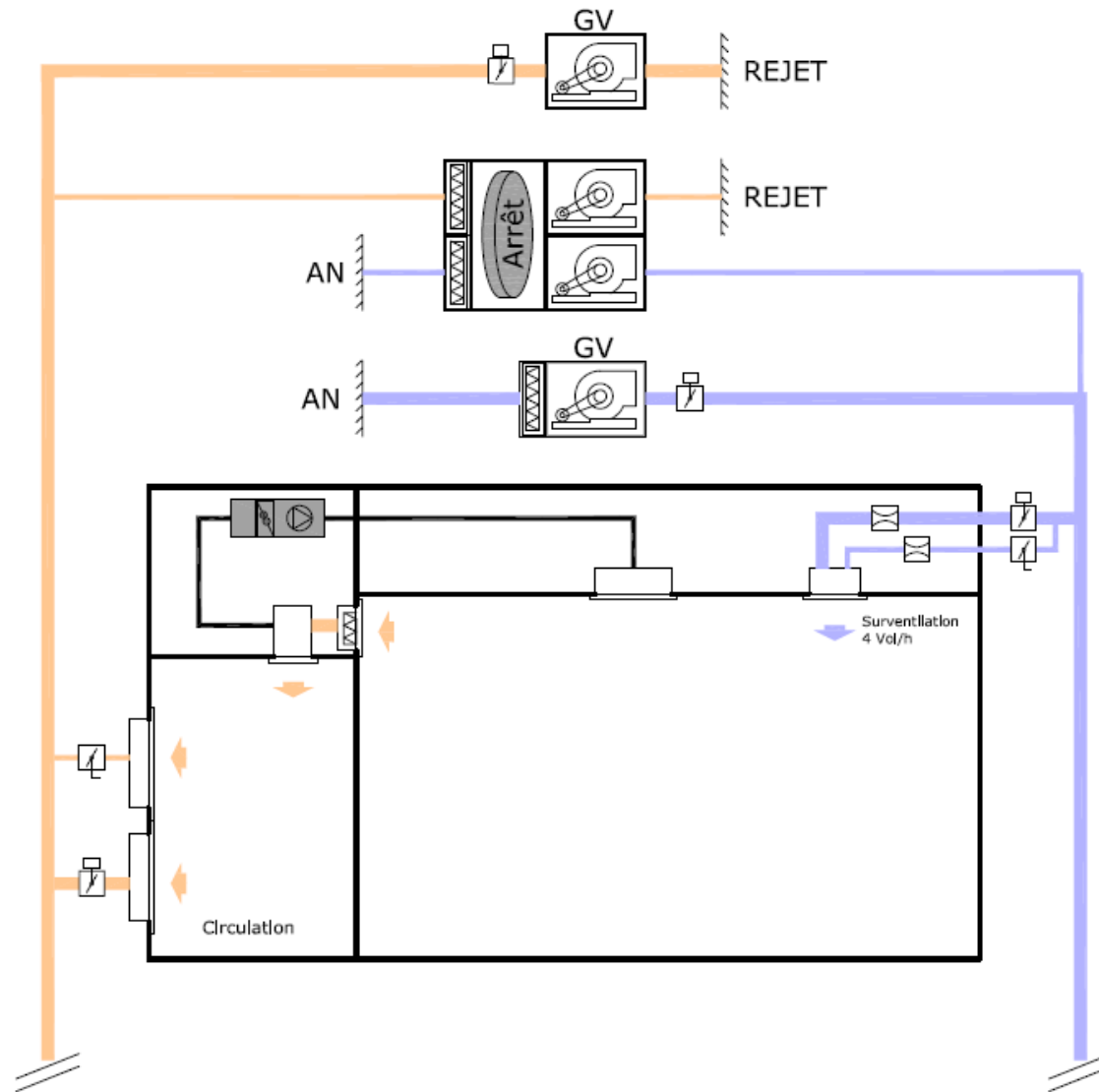
Schéma de principe aéraulique
