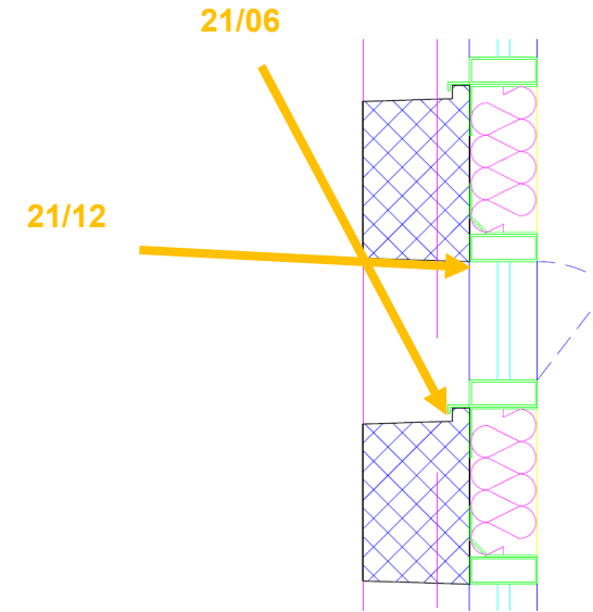
Principe de protection solaire
