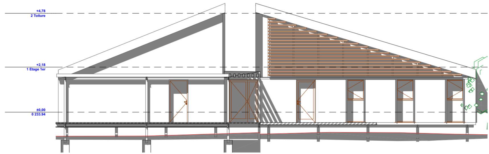
C-FS Cantine - Elevation Sud 1:50
