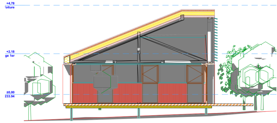
C-CA Cantine - Coupe A 1:50
