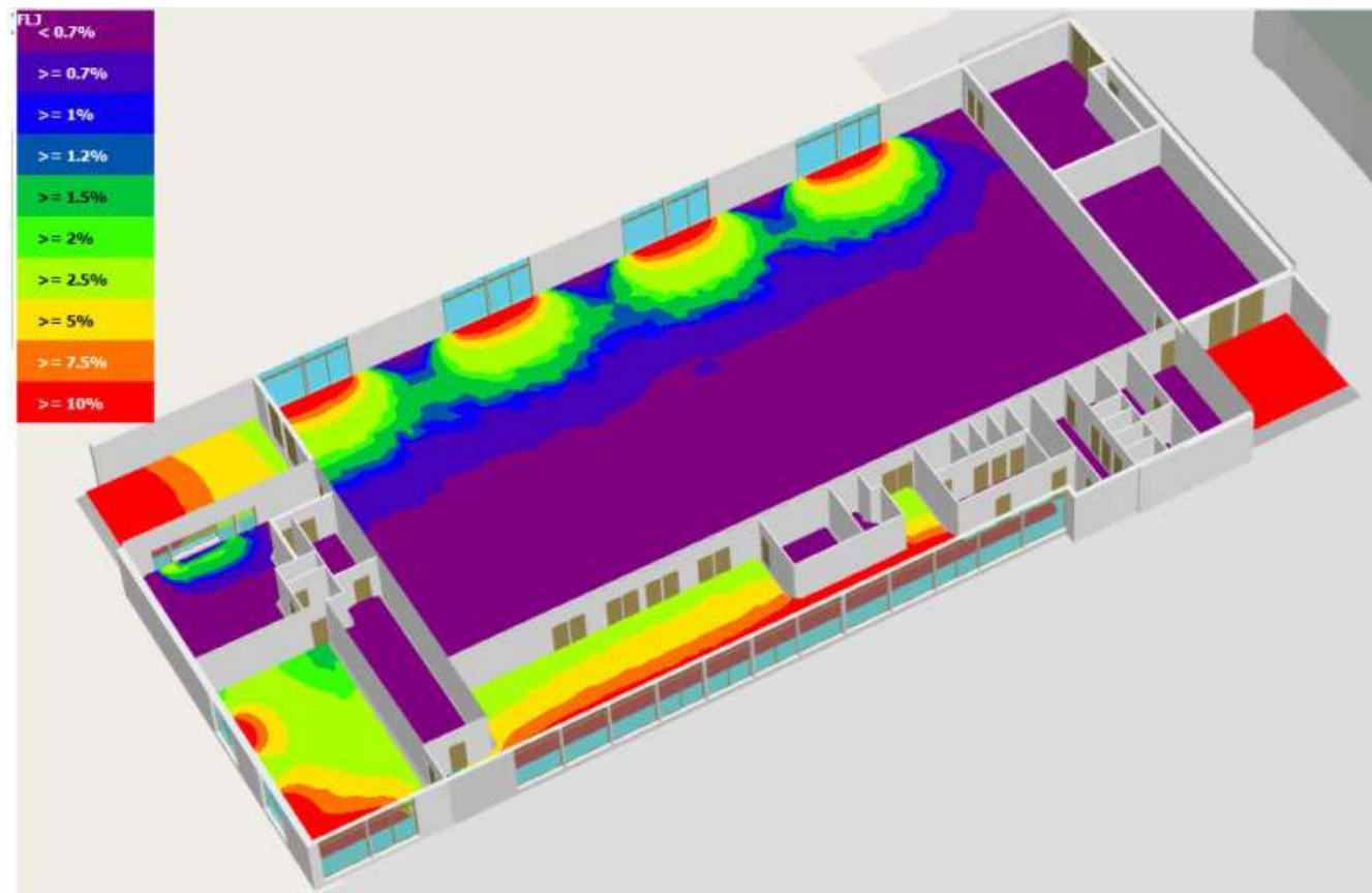
Figure 16 : Facteur Lumière du Jour - FLJ
