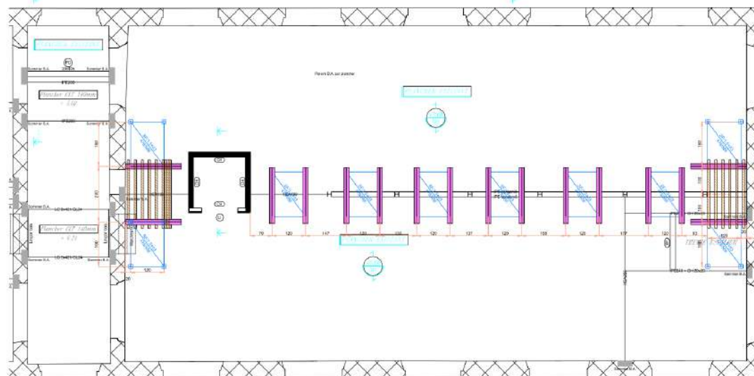
▲ Plan des étalements après démolition des planchers et poteaux
