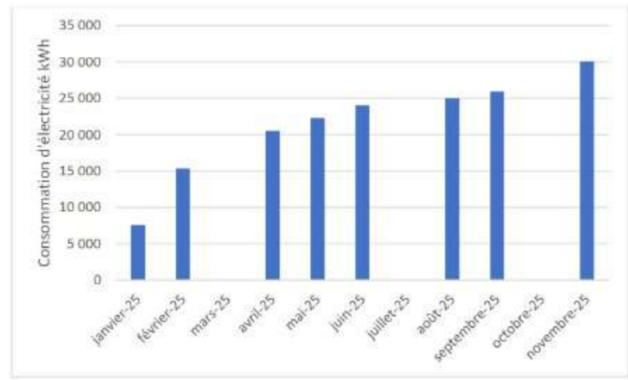
Figure 2: Consommation d'électricité au cours du chantier
