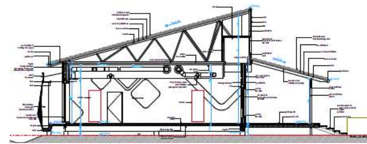
Coupe NO-SE
