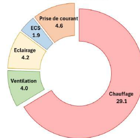
Répartition de la consommation énergétique [kWh/m²]
