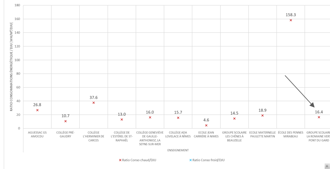
ANALYSE DES CONSOMMATIONS ÉNERGÉTIQUE PAR RAPPORT À LA RIGUEUR CLIMATIQUE [WH/M²/DJU]
